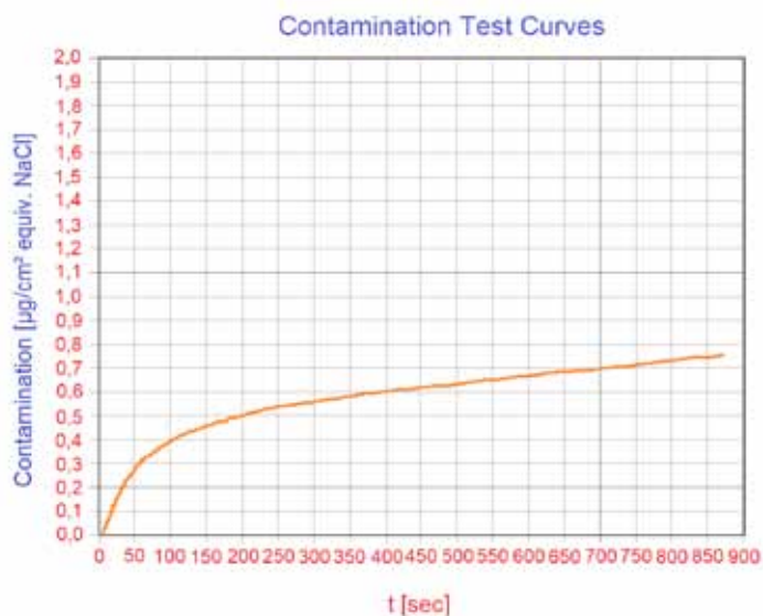
Abb. 106: Messkurve
