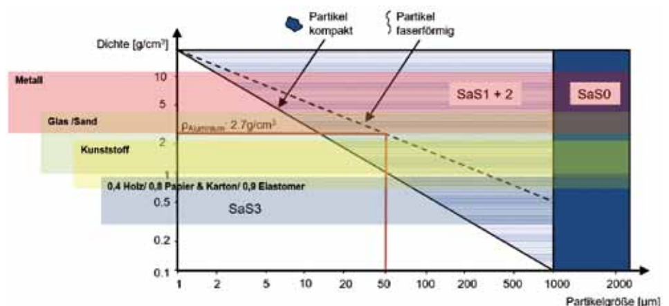
Abb. 79: Flugfähigkeitsdiagramm
