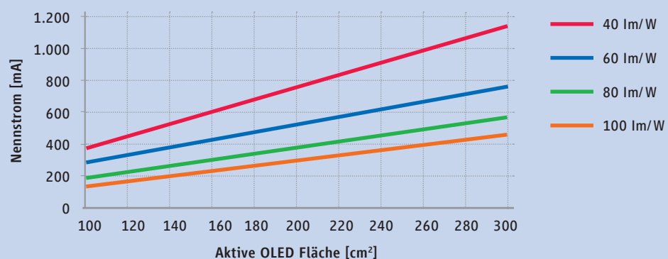
Abb. 7: Nennstromsimulation verschiedener OLEDs bei verschiedenen Flächen und Effizienzen [lm/W] (spezifische Lichtausstrahlung: 9000 lm/m 2 , Spannung 6 V)
