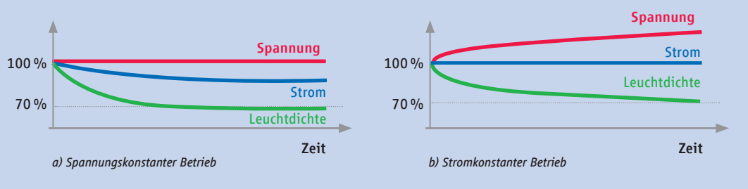
Abb. 6: Alterungsverhalten einer OLED in Abhängigkeit von Spannung und Strom
