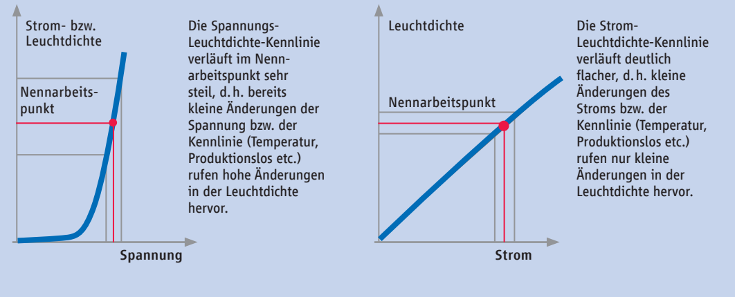
Abb. 5: Strom-Spannungs-Leuchtdichte-Kennlinien einer OLED
