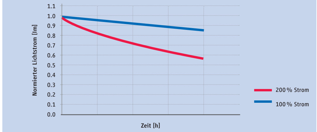
Abb. 4: Lichtstrom gegen Zeit
