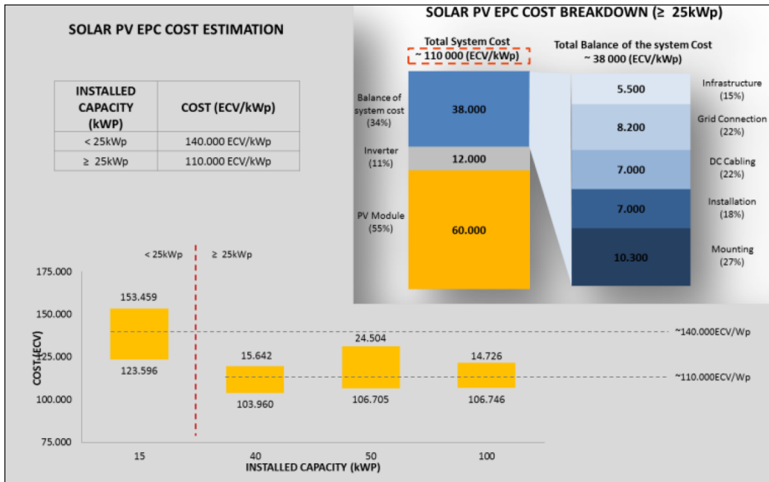
Abbildung 18: Kostenschätzung und -aufgliederung des PV-Systems in einem Hotel auf Kap Verde
