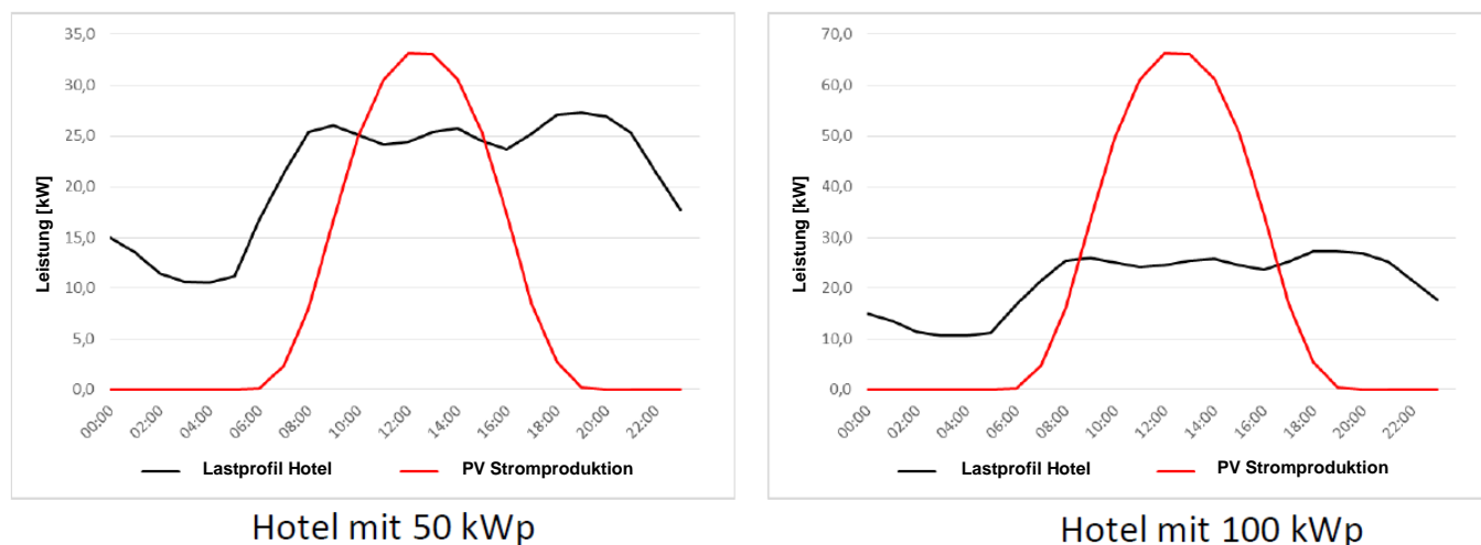
Abbildung 17: Sonneneinstrahlung und Stromproduktion zweier Hotels (50 und 100 kW)
