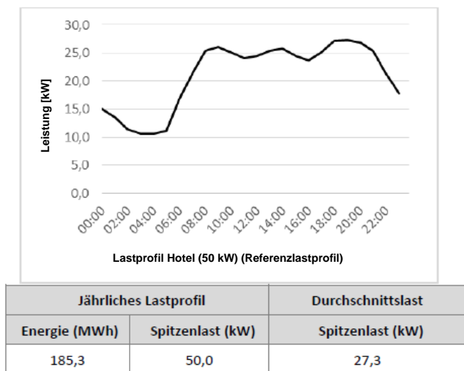
Abbildung 16: Jährlicher Strombedarf und Lastprofil eines Hotels (50 kW)
